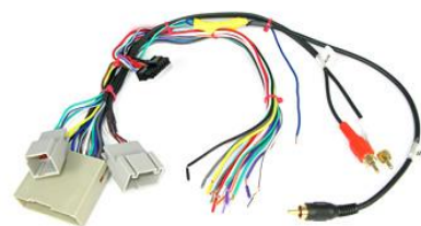
SOOFD-27 HARNESS
